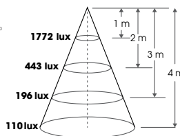
LƯỚI ĐỘ RỌI
